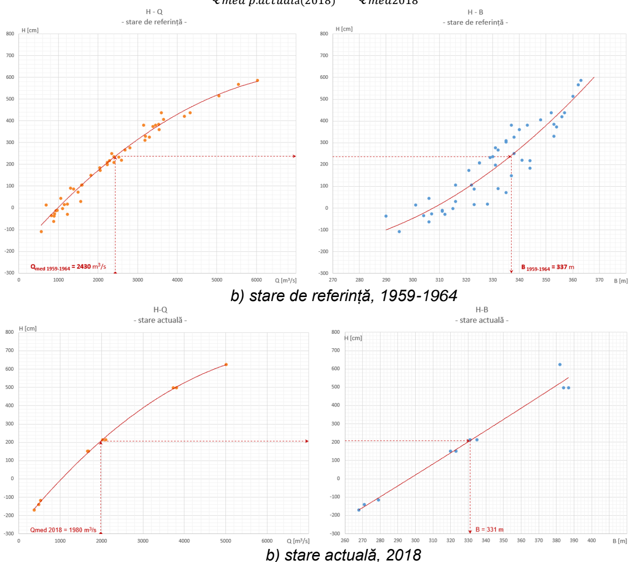
Figura C3.3.7 - Grafice cu legături corelative între nivel - debit și nivel - lățime stația hidrometrică Cernavodă
