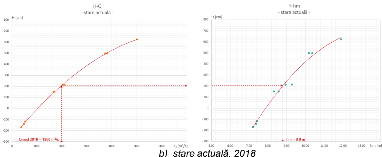
Figura C3.3.5 - Grafice cu legături corelative între nivel - debit și nivel – adâncime medie stația hidrometrică Cernavodă
