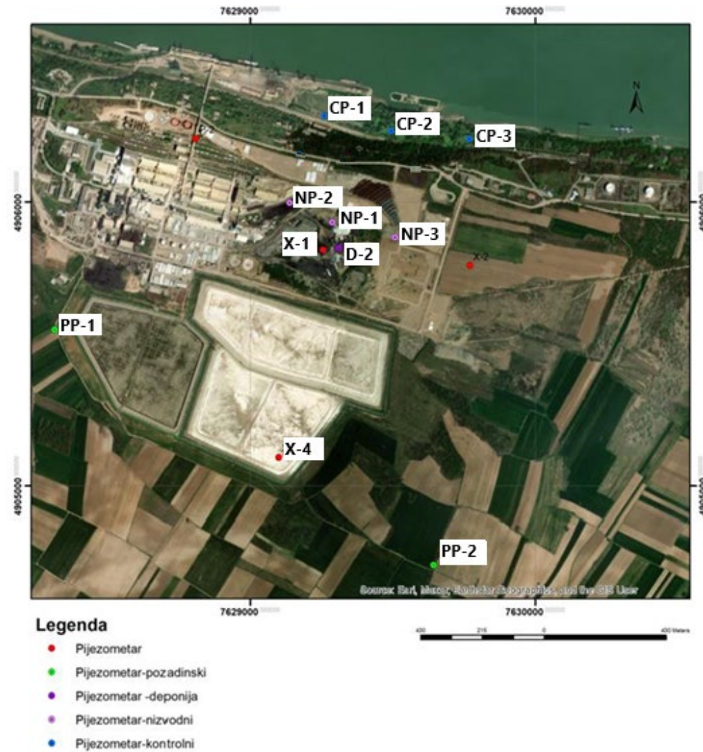
Imaginea 9.7.2 Propunere de cadru pentru amenajarea piezometrelor pentru monitorizare
