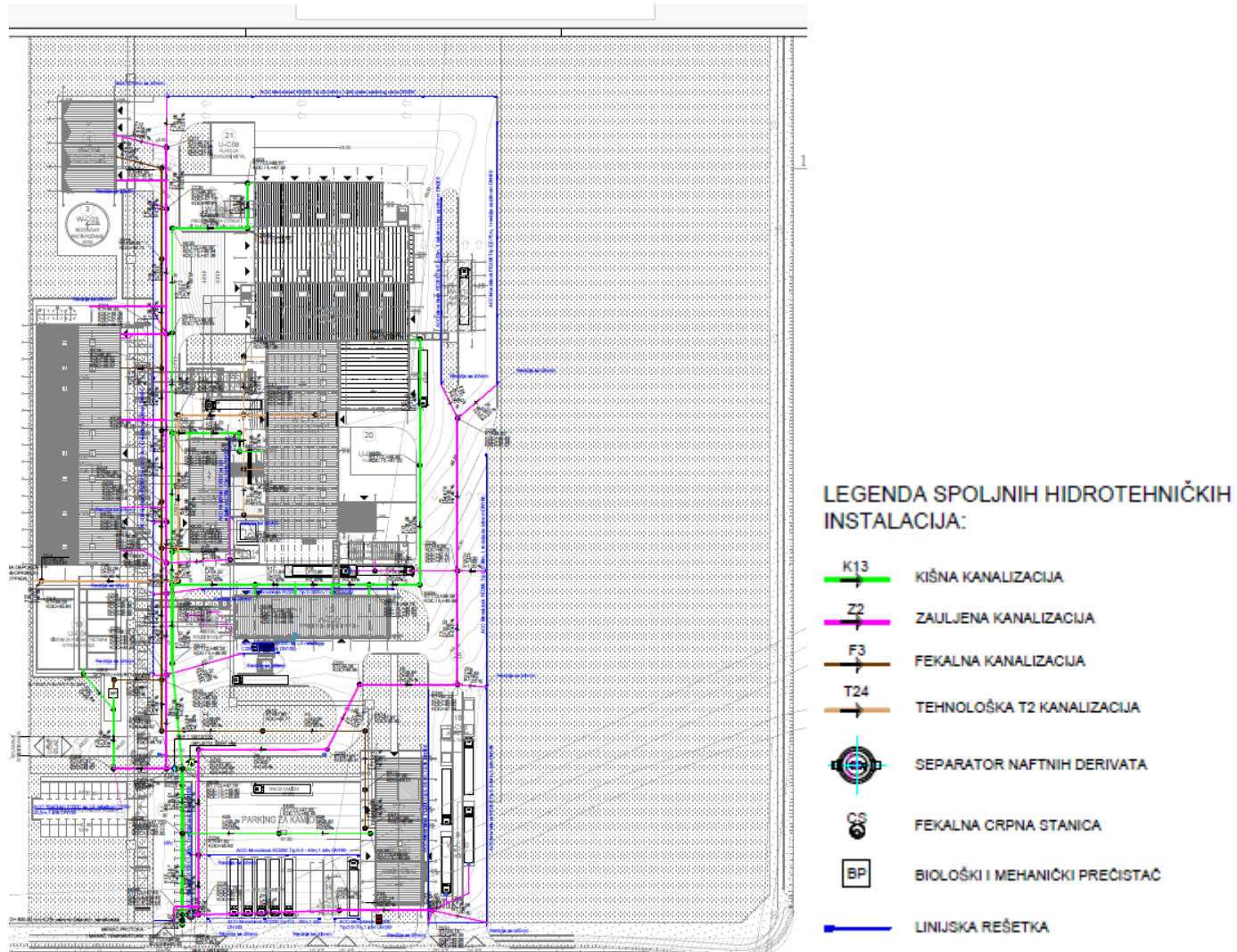
Imaginea 9.5 Situația instalațiilor hidrotehnice de canalizare
