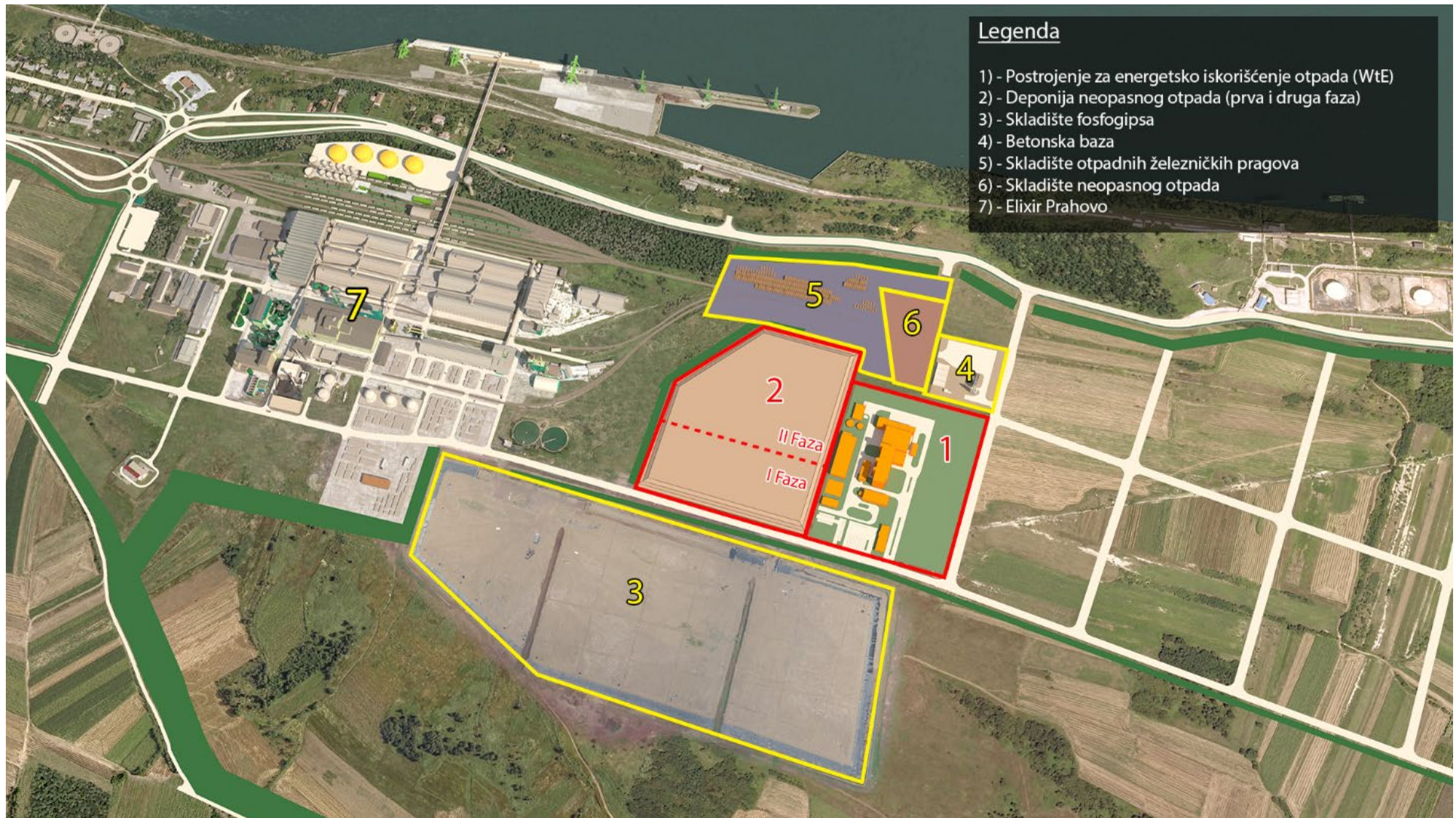
Imaginra 2.3 Microlocația uzinei pentru utilizarea energetică a deșeurilor și groapa de gunoi de deșeuri nepericuloase
