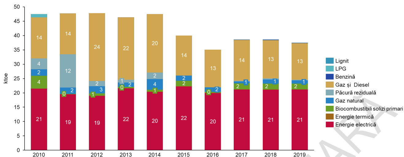
Figura 93. Evoluția consumului final de energie din industria minieră în perioada 2010-2019 (ktoe)
