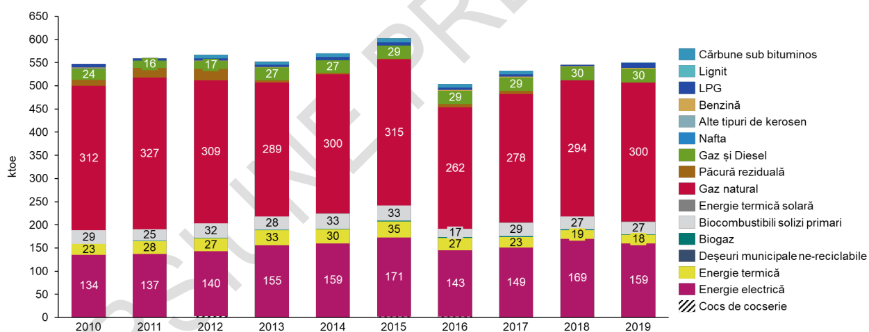
Figura 94. Evoluția consumului final de energie din industria alimentară și a tutunului în perioada 2010-2019 (ktoe)
