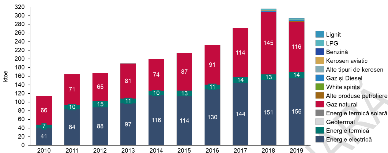
Figura 91. Evoluția consumului final de energie din industria echipamentelor de transport în perioada 2010-2019 (ktoe)
