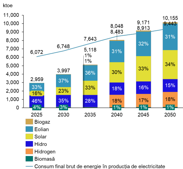
Figura 22. Evoluția ponderii SRE-E per tip de combustibil conform scenariului RO Neutră
