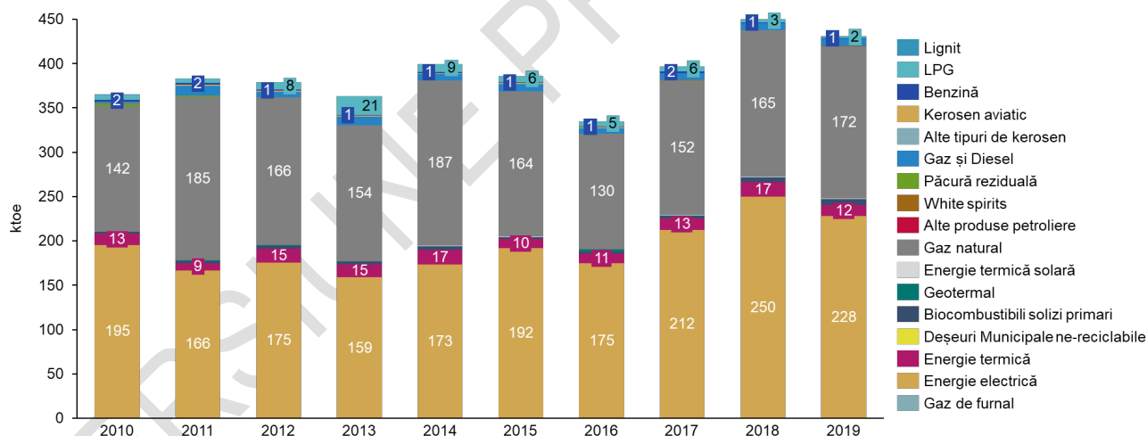
Figura 92. Evoluția consumului final de energie din industria utilajelor în perioada 2010-2019 (ktoe)
