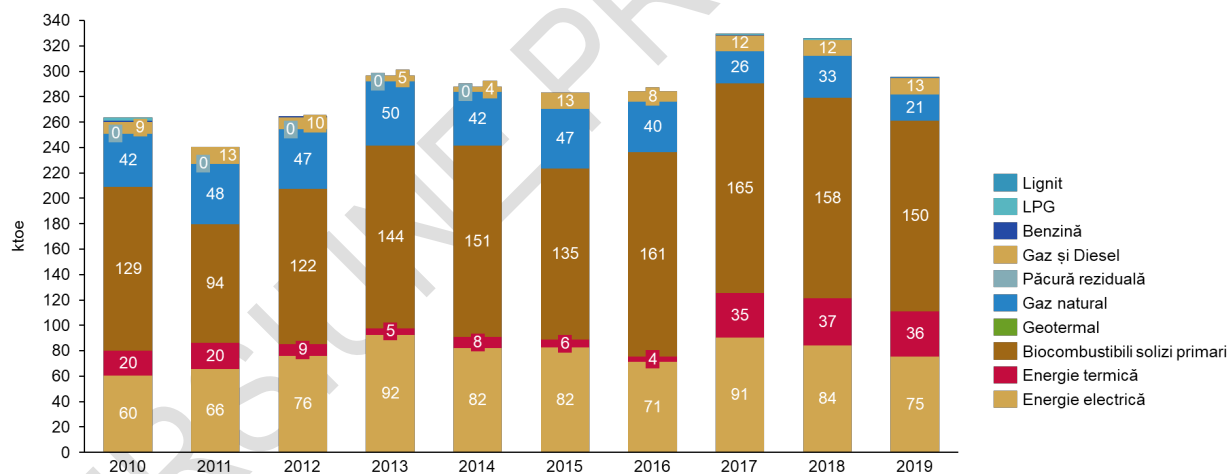
Figura 96. Evoluția consumului final de energie din industria lemnului și a produselor din lemn în perioada 2010-2019 (ktoe)
