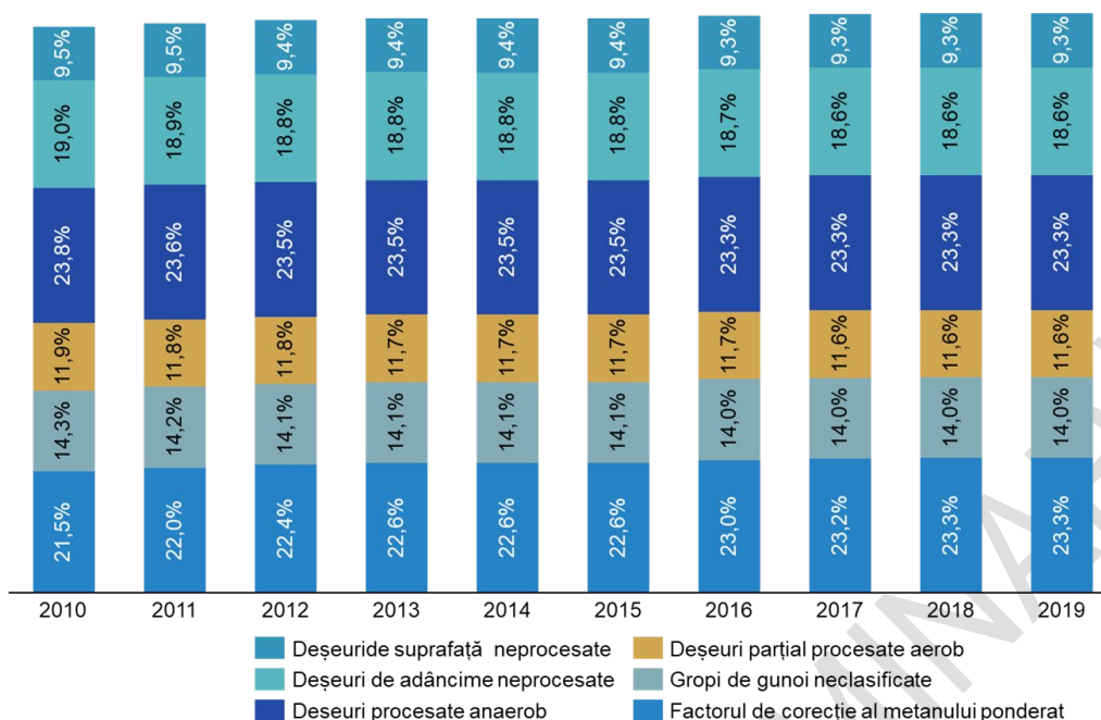
Figura 117. Factorul de corecție al metanului în industrie
