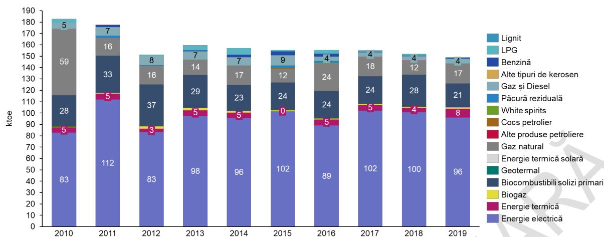
Figura 99. Evoluția consumului final de energie din domeniul alte industrii în perioada 2010-2019 (ktoe)
