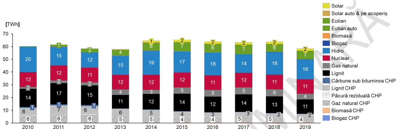
Figura 64. Evoluția producției de energie electrică a centralelor electrice și în CHP în perioada 2010 - 2019 (mii GWh)
