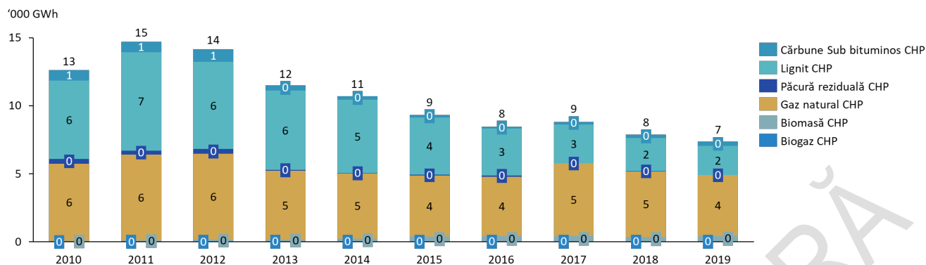
Figura 71. Evoluția producției de energie electrică a centralele în cogenerare în perioada 2010-2019 (GWh)
