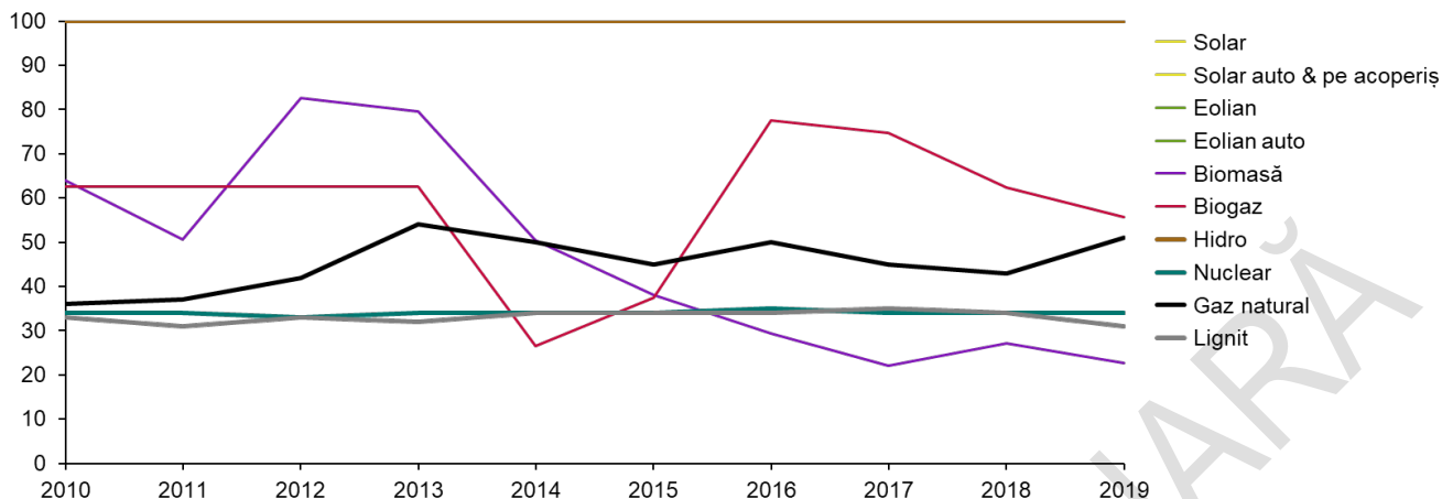
Figura 69. Eficiența capacităților de producție a energiei electrice per tehnologie în perioada 2010-2019 (%)
