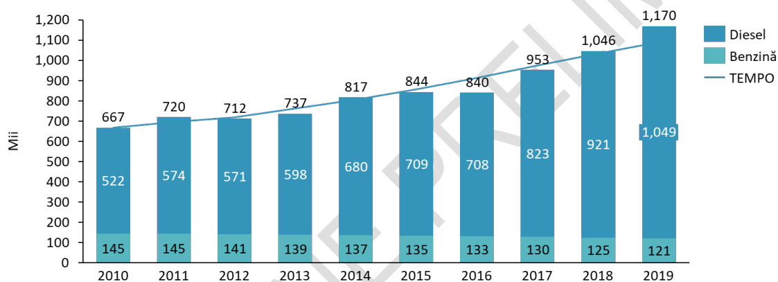
Figura 78. Evoluția numărului de autovehicule transport marfă în perioada 2010-2019 conform INS și clasificarea lor pe tip de combustibil conform LEAP_RO
