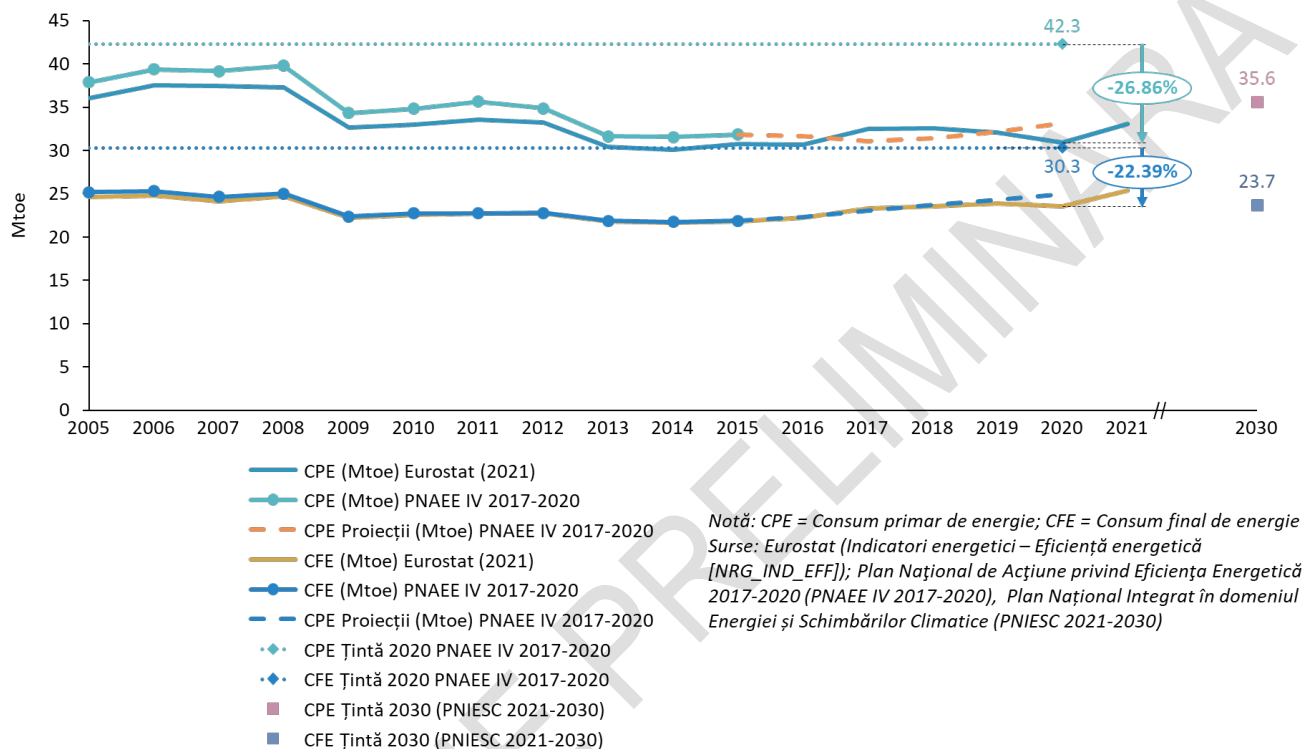
Figura 24. Tendință istorică în EE
