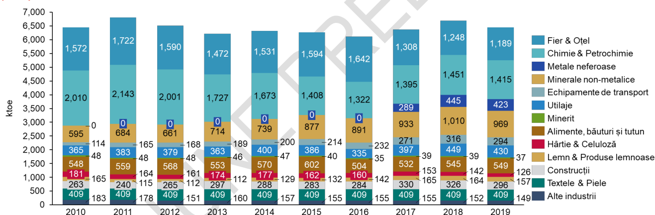
Figura 86. Evoluția consumului final de energie în sectorul Industrie în perioada 2010-2020 per domeniu industrial (ktoe)
