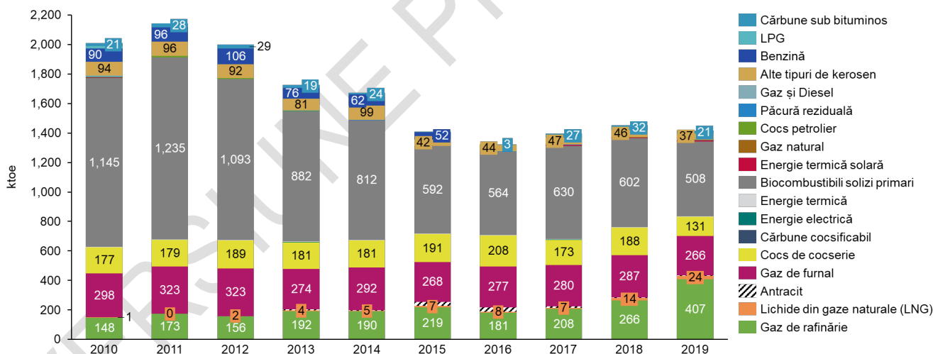
Figura 88. Evoluția consumului final de energie din industria chimică și petrochimică în perioada 2010-2019 (ktoe)
