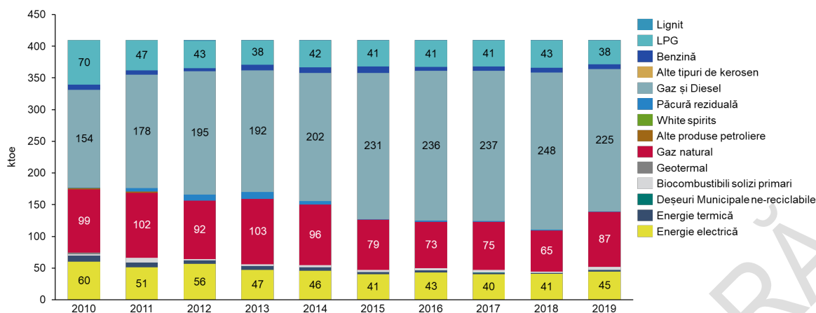
Figura 97. Evoluția consumului final de energie din industria construcțiilor în perioada 2010-2019 (ktoe)
