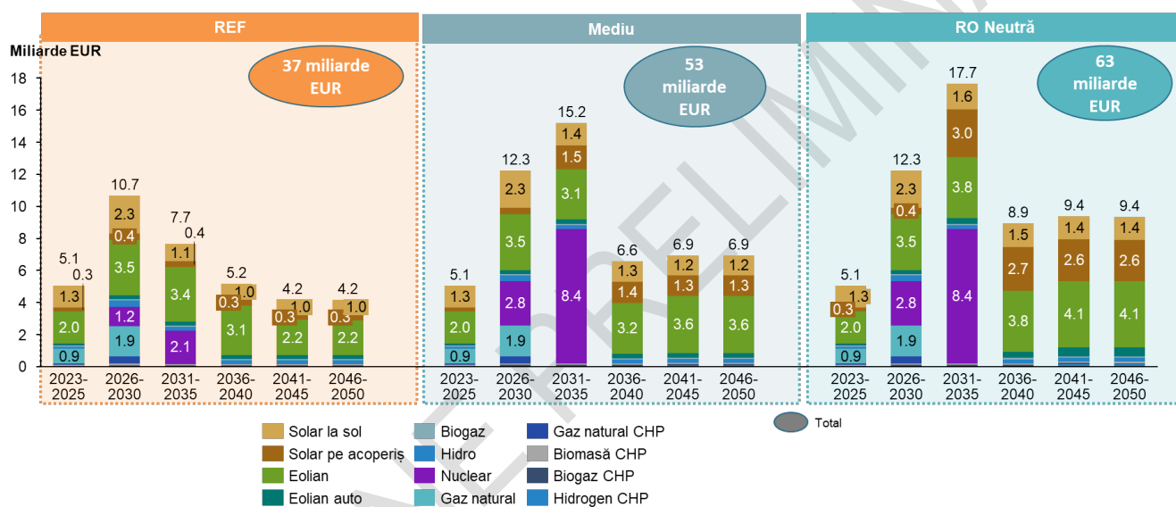
Figura 51. Valoarea totală a investițiilor necesare până în 2050 în domeniul producției de energie electrică conform celor 3 scenarii
