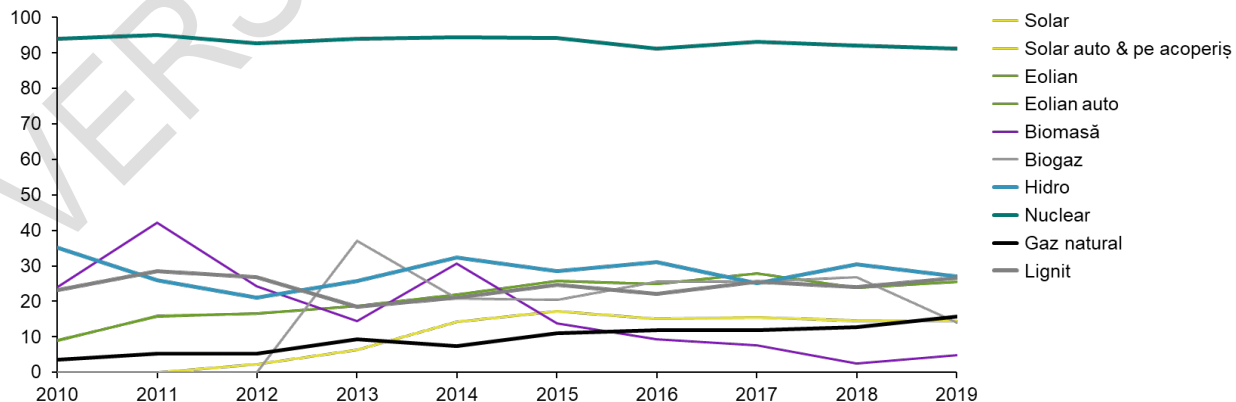
Figura 68. Disponibilitatea capacităților de producție a energiei electrice în perioada 2010-2019 (%)
