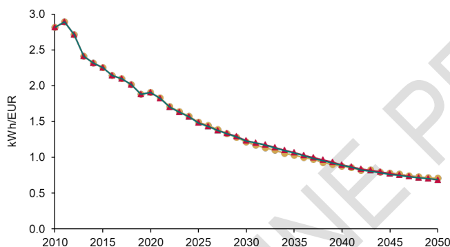
Figura 57. Intensitatea energetică primară - Consumul primar de energie raportat la PIB
