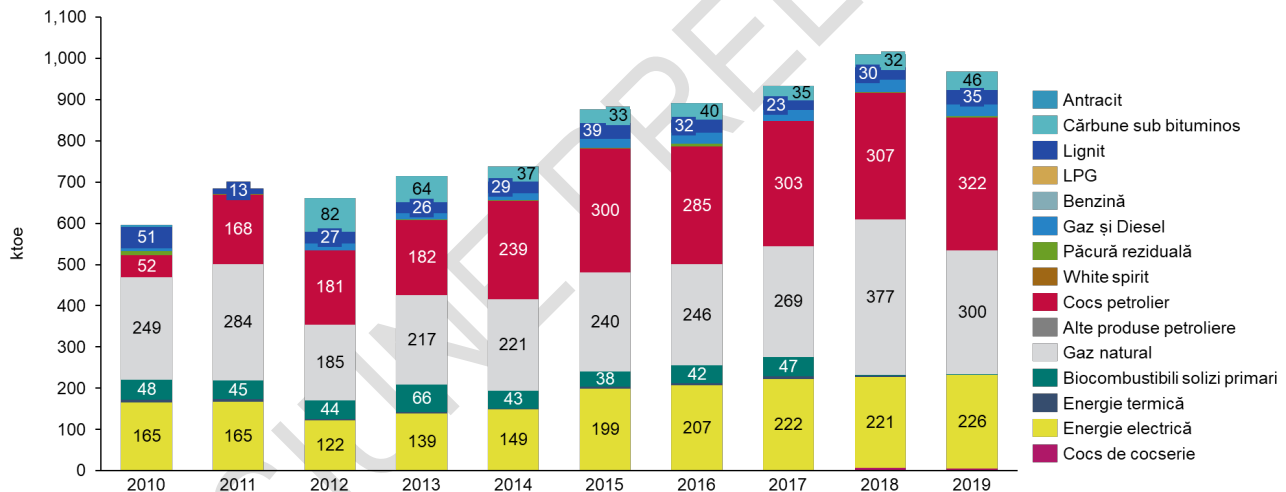
Figura 90. Evoluția consumului final de energie din industria mineralelor nemetalice în perioada 2010-2019 (ktoe)
