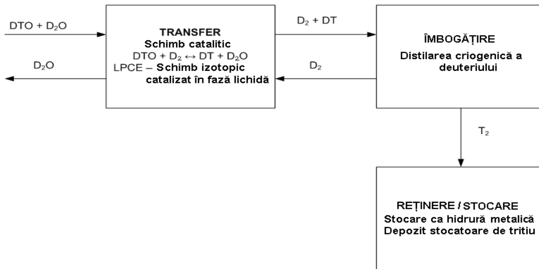
Figura 3.2 Schema simplificată de proces al Proiectului CTRF
