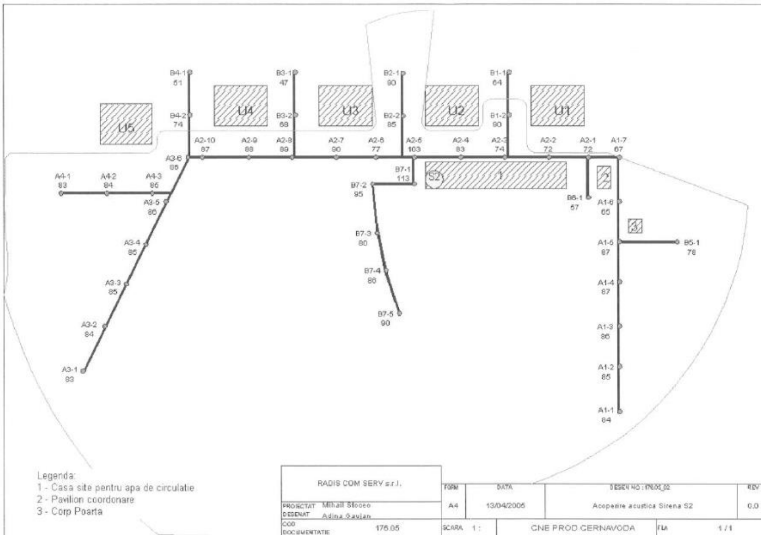
Figura nr. 5.6. Schema acoperirii acustice Sirena - S2
