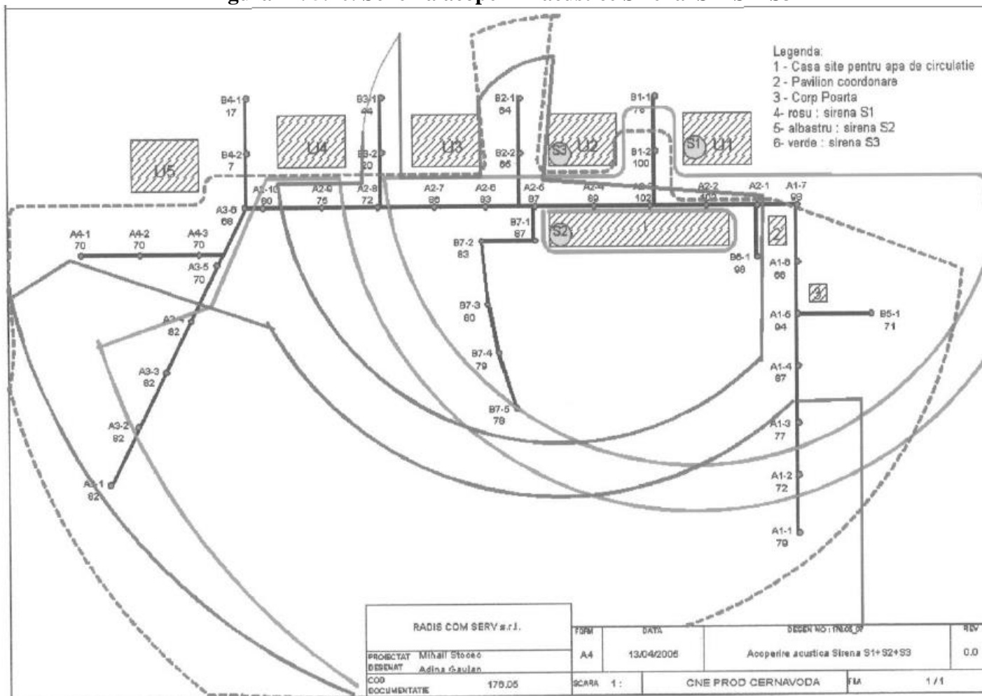
Figura nr. 5.10. Schema acoperirii acustice Sirena S1+S2+S3
