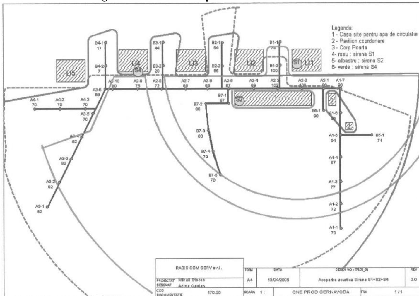
Figura nr. 5.11. Schema acoperirii acustice Sirena S1+S2+S4
