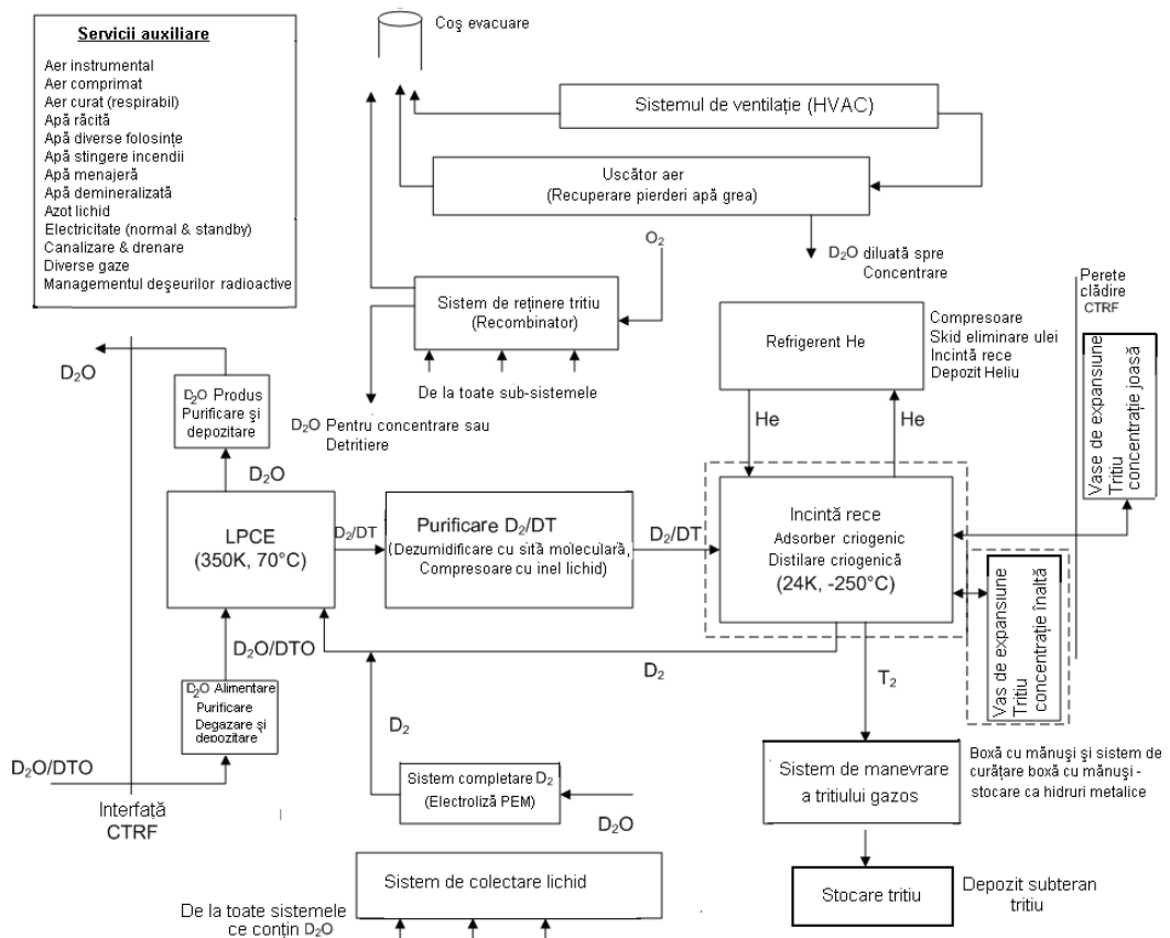
Figura 3.1 Schema bloc a instalației CTRF
