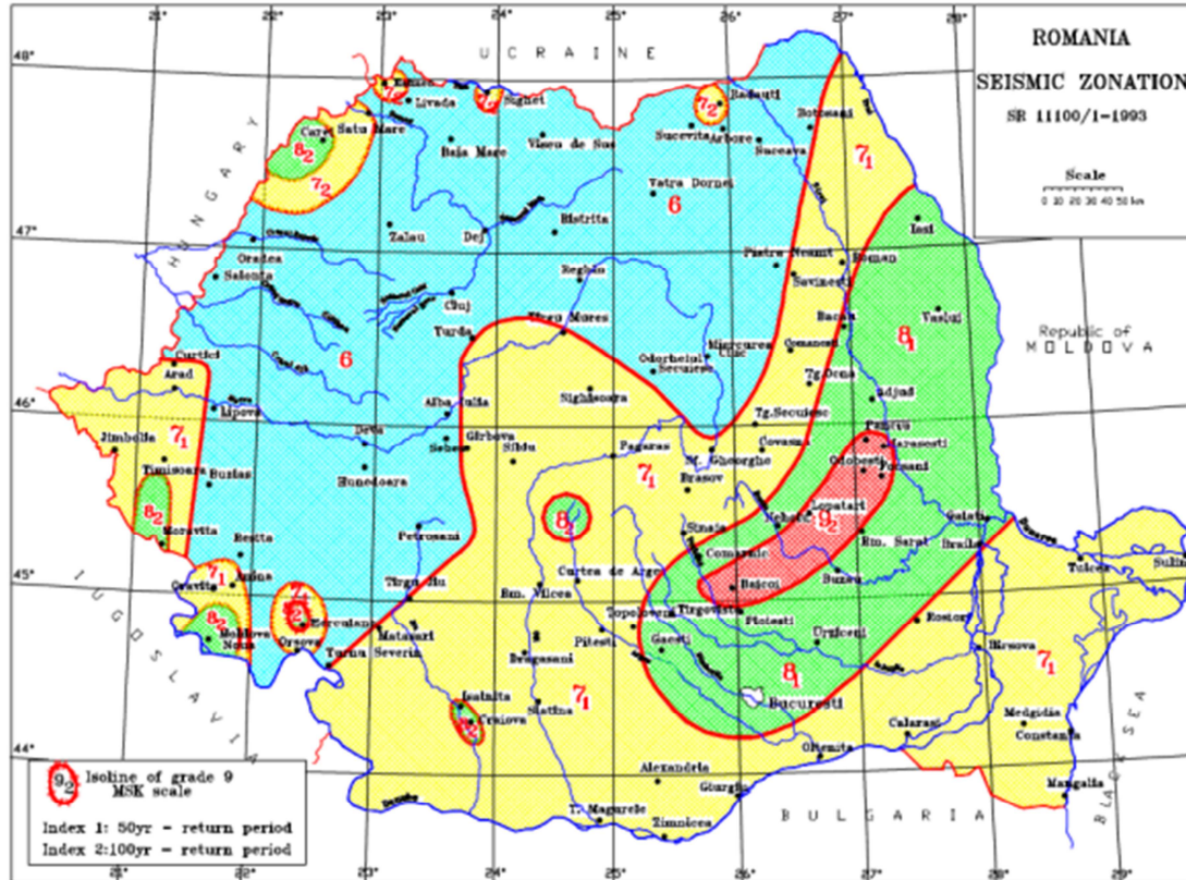
Figura nr. 2.7. Zonarea seismică (STAS 11 100/93)
